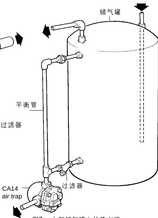
图7：小型储气罐上的疏水阀
