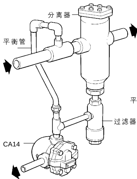
图6：压缩空气主管的汽水分离器上应用的疏水阀
